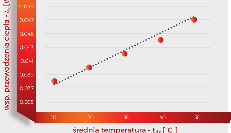
Zmiana wsp. przewodzenia ciepła w zależności od średniej temperatury
