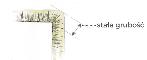
Mata lamelowa - prostopadły układ włókien
